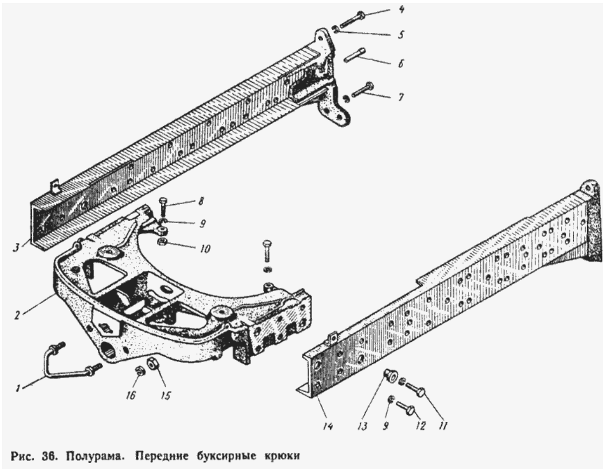
Рис. 36. Полурама. Передние буксирные крюки.
